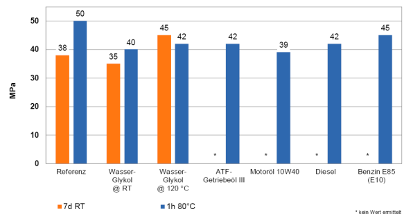
Druckscherfestigkeit nach Medieneinlagerung für 1000 h, DELO Norm 5
