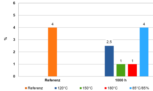
Reißdehnung nach Temperaturlagerung, in Anlehnung an DIN EN ISO 527 Aushärtung: 1h +80°C
